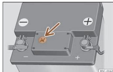
Abb. 233 Sichtfenster an der Oberseite der 12-Volt-Fahrzeugbatterie (Prinzipdarstellung).
