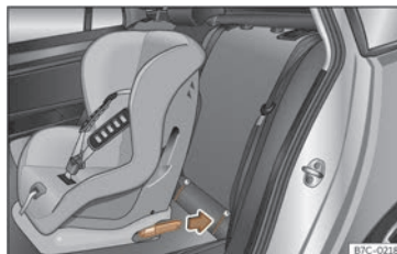
Abb. 42 Rückseite: Einbau des Kindersitzes mit dem ISOFIX-System.
