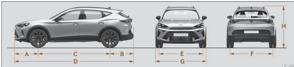
Abb. 251 Abmessungen
