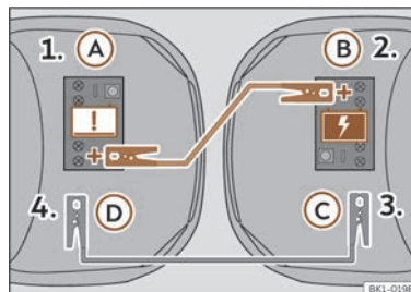
Abb. 210 Anschlussplan der Starthilfekabel.
