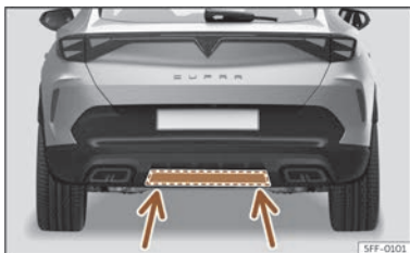
Abb. 87 Erfassungsbereich des unteren Sensors
