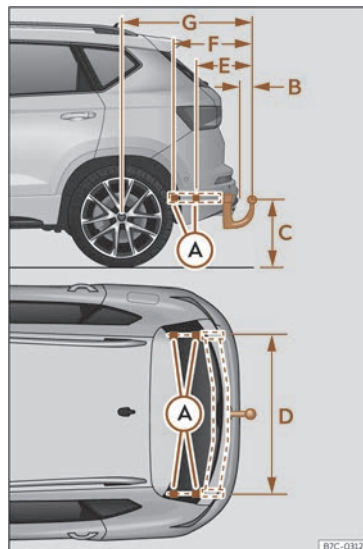
Abb. 179 Maße und Befestigungspunkte für den nachträglichen Einbau einer Anhängervorrichtung
