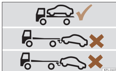
Abb. 188 Mit einem Abschleppfahrzeug transportieren: Fahrzeuge mit automatischem Getriebe und Allradantrieb (4Drive).
