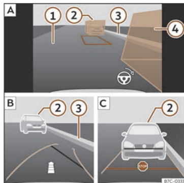
Abb. 140 Anzeige am Bildschirm des Infotainment-Systems: Rückfahrasistent, Modus 2.
