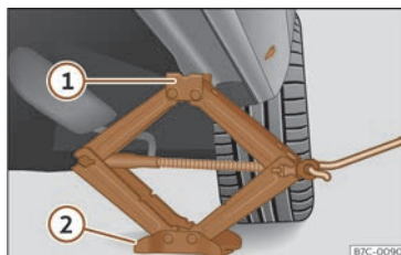
Abb. 217 Längsträger: Wagenheber ansetzen.
