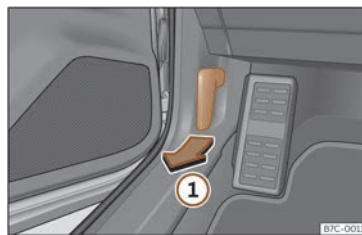
Abb. 197 Entriegelungshebel im Fahrerfußraum.
