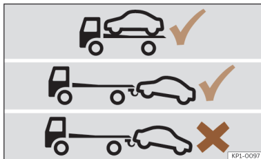
Abb. 187 Mit einem Abschleppfahrzeug transportieren: Fahrzeuge mit automatischem Getriebe und Frontantrieb.
