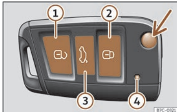
Abb. 41 Fahrzeugschlüssel für das Fahrzeug.
