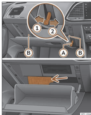
Abb. 194 Rechtslenker: Abdeckung des Sicherungskastens an der Instrumententafel, Beifahrerseite.
